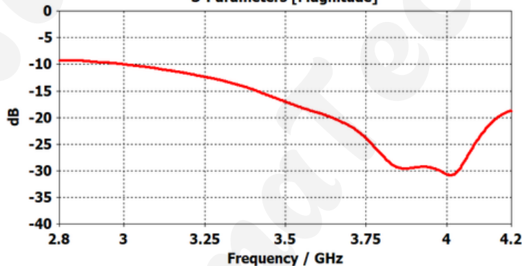
S-Parameters [Magnitude]
